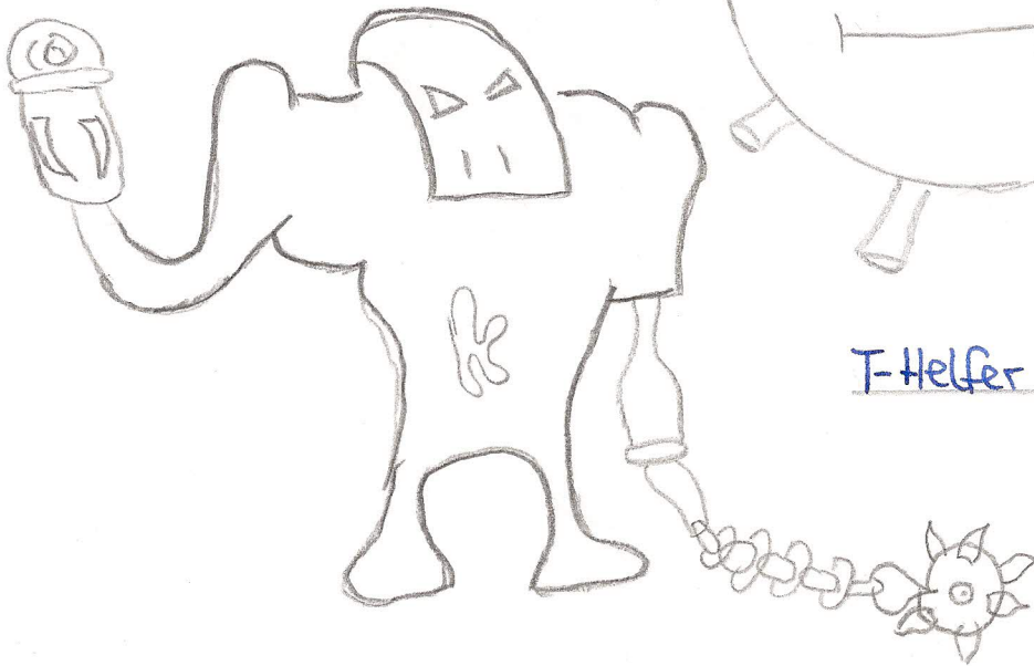
killer Zelle
